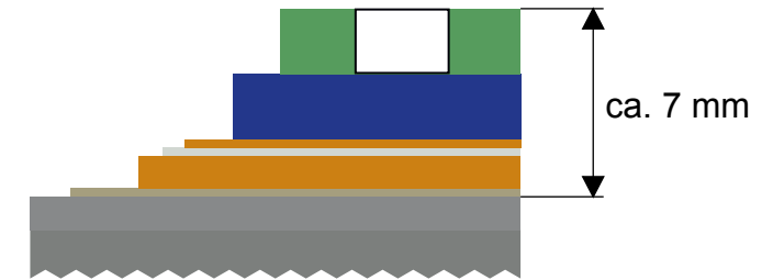
Systemaufbau
